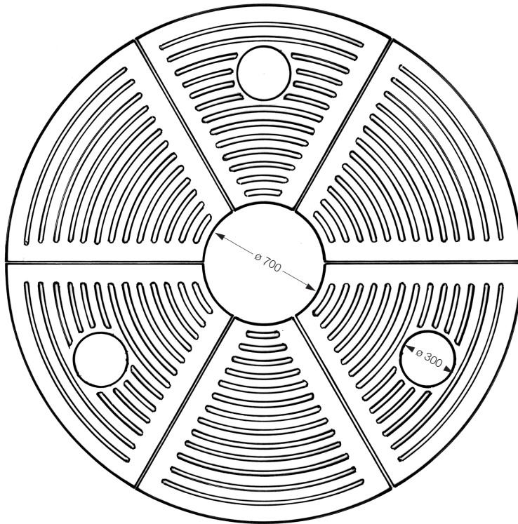
Baumroste BR 004
